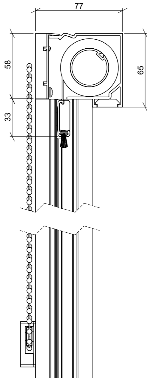
SECTION A-A
